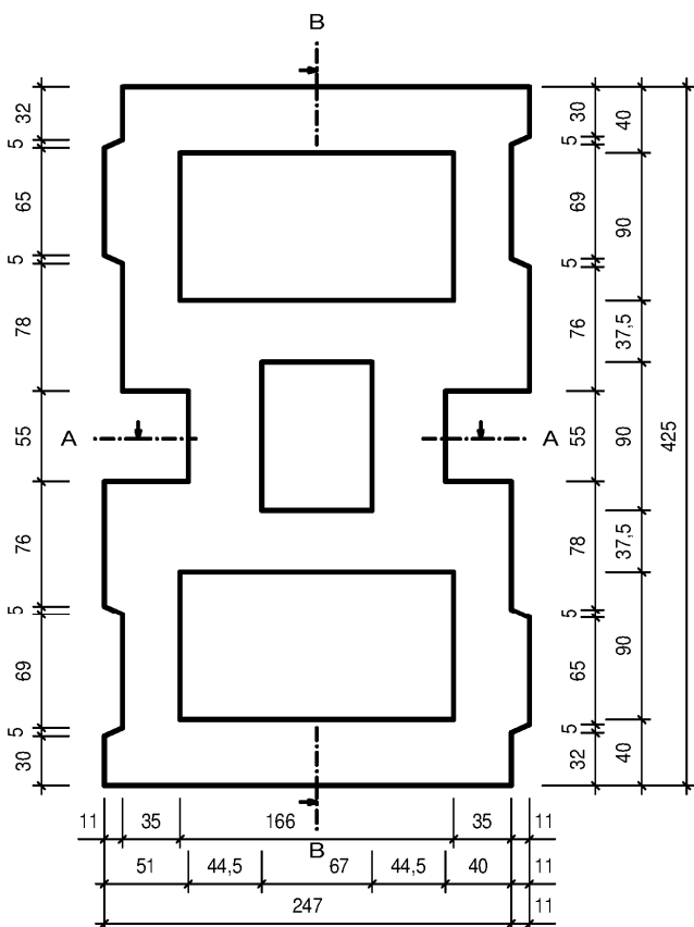
Untersicht
